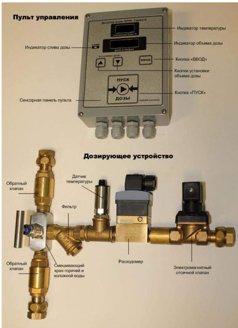
Рис 1: Общий вид дозатора
