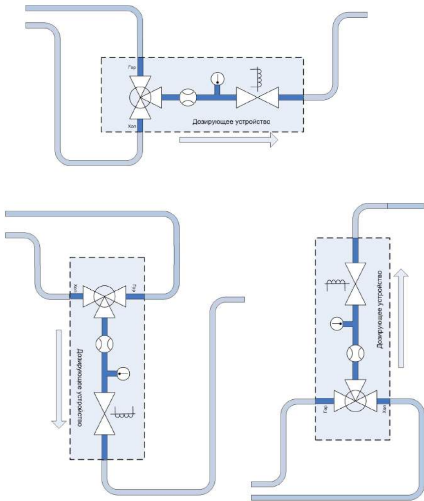
Рис 3: Правильное подключение
