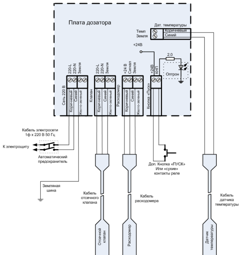
Рис 7: Монтажная схема дозатора
