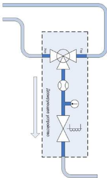
Рис 4: Неправильное подключение
