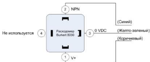
Рис 8: Подключение расходомера
