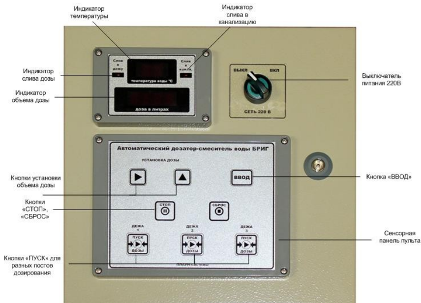
Рис 1: Пульт управления
